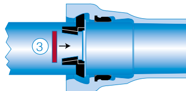
Blocage
