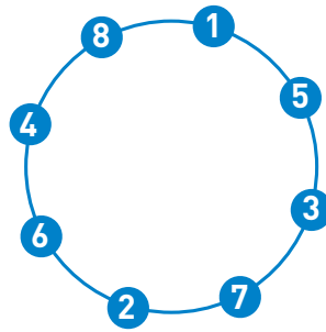
8 boulons
