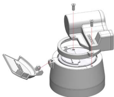
Fig. 4: Montaje del EDC-C
