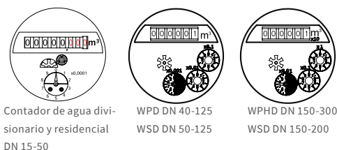
Fig. 1: Relojerías ZENNER con disco modulador
