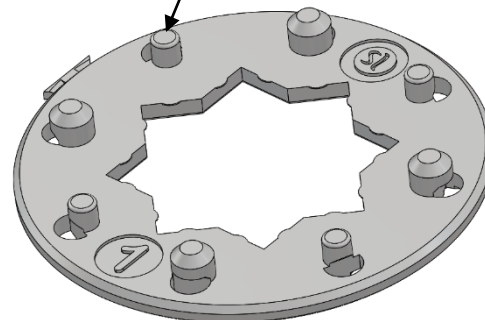
Picots de centrage de la rondelle dans le corps de tabernacle
