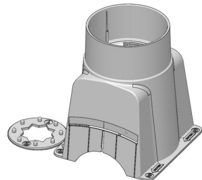
Vue du côté abonné
