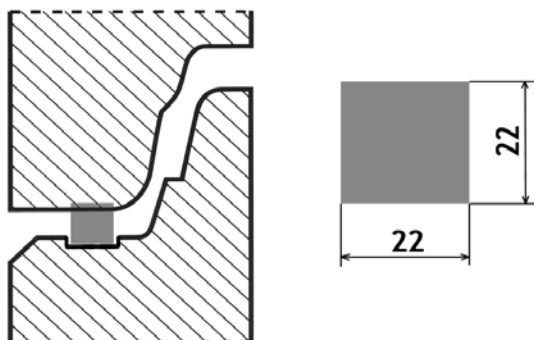
Section carrée
