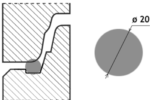
Section ronde
