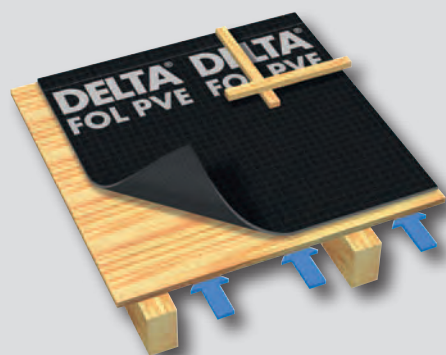
Support continu ventilé en sous-face.
