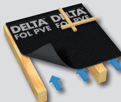
Support discontinu (écran de sous-toiture ventilé en sous-face).
