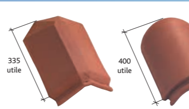
About d'arêtier angulaire à emboîtement Réf. 859 About d'arêtier 1/2 rond à emboîtement grand modèle Réf. 851 (5)
