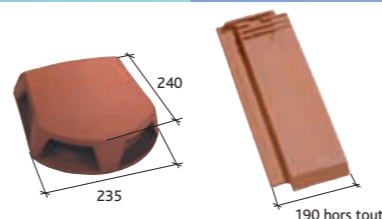
Lanterne bi-section Ø 126 utile et Ø 160 utile (Section aération: 130 cm 2 ) (conforme VMC) Réf. 1000 1/2 tuile Alpha 10 Réf. 200.01
