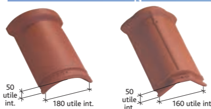
Faitière/arêtier 1/2 rond à emboîtement petit modèle (3 au ml) Réf. 700 (2) Crochet adapté: crochet F6-Réf. CRP 700/706 Faitière/arêtier grand modèle à emboîtement (3 au ml) Réf. 706 (4) Crochet adapté: crochet F6-Réf. CRP 700/706
