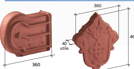
About de rive universelle droit à emboîtement Réf. 1073 (2) Fronton de rive universelle Réf. 1083 (2)
