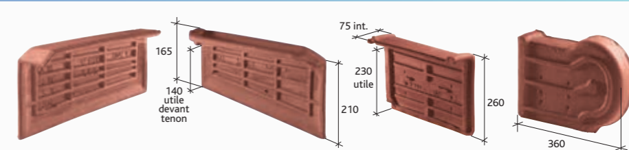
Rive individuelle gauche à recouvrement (2,7 par ml au pureau de 375 mm) Réf. 200.42 (1) Rive individuelle droite à emboîtement (2,7 par ml au pureau de 370 mm) Réf. 200.41 (1) Rive universelle (3 au ml) Réf. 1051 (2) About de rive universelle gauche à recouvrement Réf. 1072 (2)
