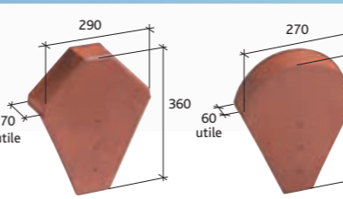
Fronton pour faitière angulaire à emboîtement Réf. 801 Fronton petit modèle pour faitière 1/2 ronde et faitière conique (petite ouverture) Réf. 803 (3)
