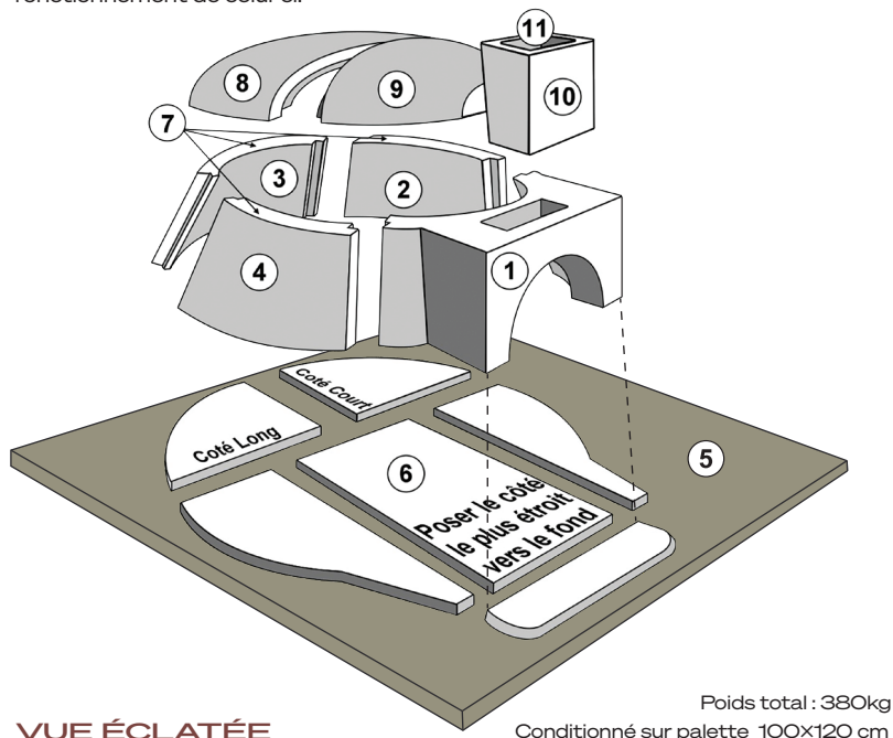
VUE ÉCLATÉE
