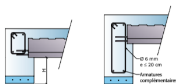
Linteaux banchés : e = écartement entre cadres
