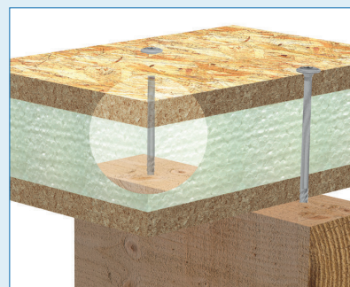
Fixation de panneaux sandwich
