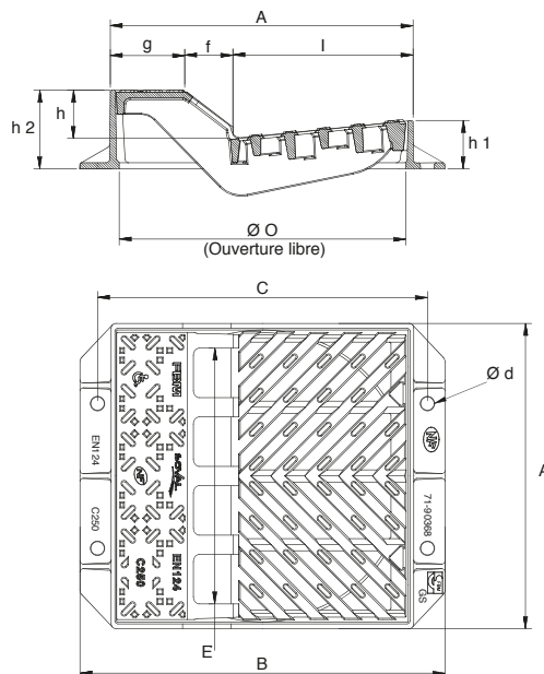
Grille avaloir profil A
