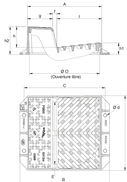
Grille avaloir profil T
