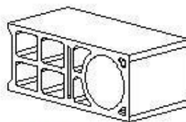
Réf. coupe demi - poteau angle
