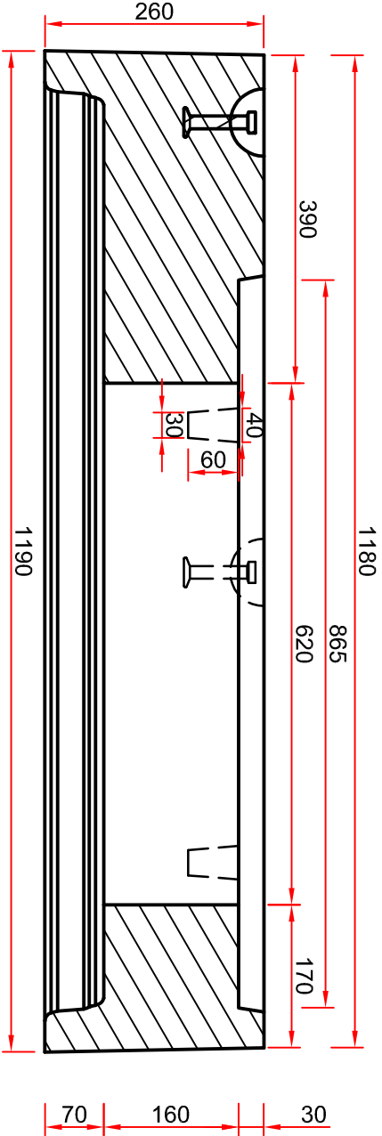
A-A (1:8)
