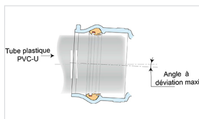
Jonction IZIFIT-K non verrouillée pour tubes plastiques
