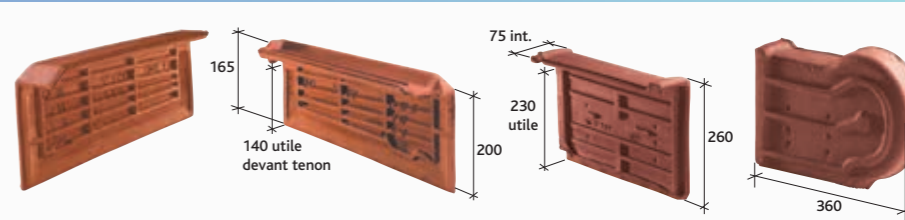
Rive individuelle gauche à recouvrement Rhôna 10 (2,6 par ml au pureau de 385 mm) Réf. 200.42 (1) Rive individuelle droite à emboîtement Rhôna 10 (2,6 par ml au pureau de 385 mm) Réf. 200.41 (1) Rive universelle (3 au ml) Réf. 1051 (3) About de rive universelle gauche à recouvrement Réf. 1072 (3)
