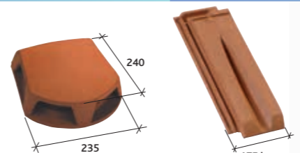
Lanterne bi-section Ø 126 utile et Ø 160 utile (Section aération : 130 cm 2 ) (conforme VMC) Réf. 1000 1/2 tuile Rhôna 10 Réf. 222.01
