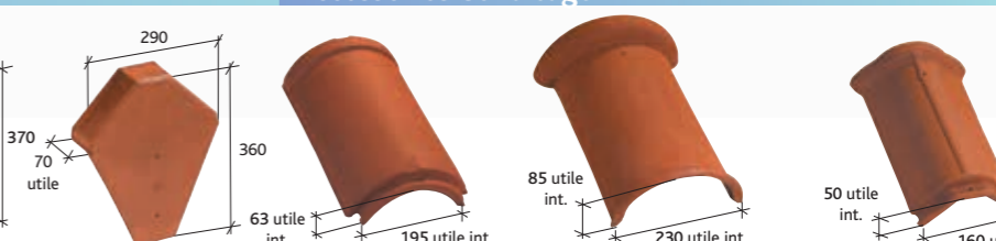
Fronton pour faîtière angulaire à emboîtement Réf. 801 Faîtière/arêtier 1/2 rond à emboîtement grand modèle (2,5 au ml) Réf. 702 (8) Crochet adapté : crochet F1-Réf. CRP 702 Faîtière à bourrelet à emboîtement (2,5 au ml) Réf. 715 (3) Crochet adapté : crochet F5-Réf. CRP 715
