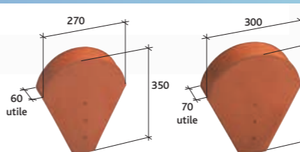
Fronton petit modèle pour faîtière 1/2 ronde et faîtière conique (petite ouverture) Réf. 803 (8) Fronton grand modèle pour faîtières lisse, à bourrelet et conique (grande ouverture) Réf. 804 (3)
