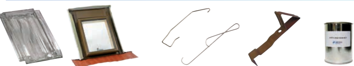
Tuile en verre Réf. VER 222 Châssis aluminium universel pour tuiles faiblement galbées, plates et à pureau plat (double vitrage) Réf. CHFACTPPP (2) Fixation dans l'emboîtement Réf. MONO 14 -17 Crochet «V1» fixation pour plain carré Réf. CRV 01 Crochet à neige Réf. CRN 14 (6)(7) Pot de Peinture 25cl pour retouches coloration Tuiles IMERYS-Coloris Ardoisé Réf. PEINT01
