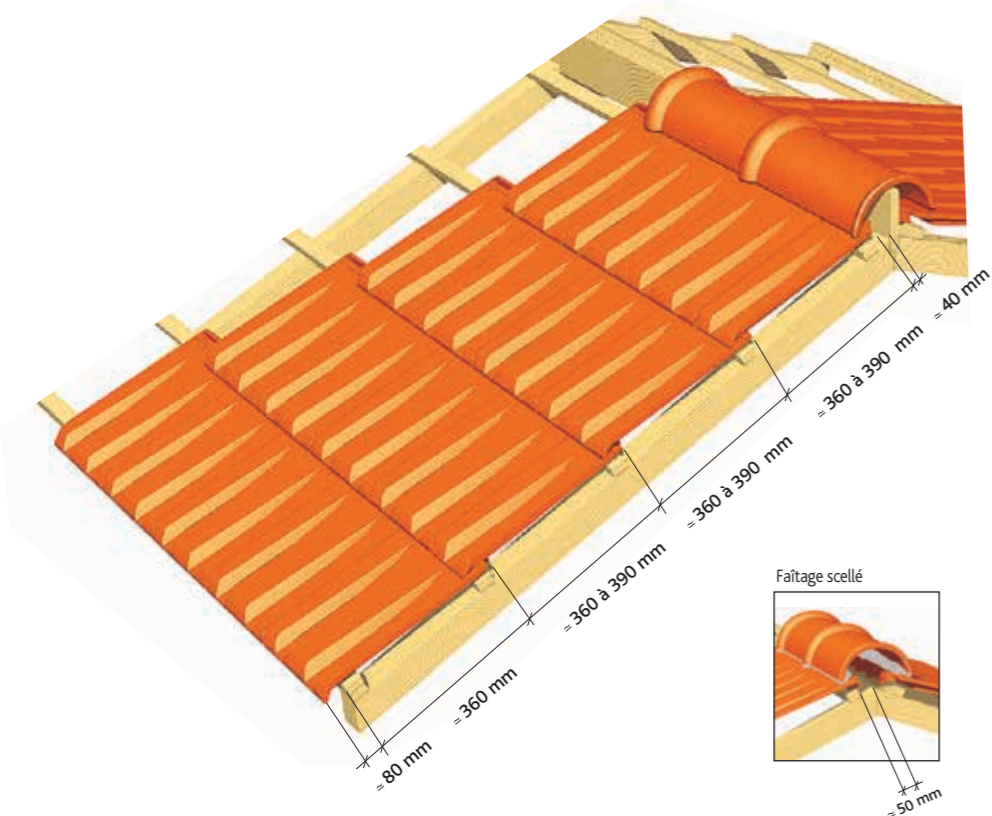
Faîtière / arêtier angulaire à emboîtement (3 par ml) Réf. 710 Crochet adapté : crochet F3-Réf. CRP 705 About d'arêtier 1/2 rond à emboîtement grand modèle Réf. 851 (8) About d'arêtier grand modèle à emboîtement Réf. 854 (3) About d'arêtier angulaire à emboîtement Réf. 859 Rencontre porte poinçon petit modèle 3 ouvertures angulaires Réf. 903 (3) Rencontre porte poinçon petit modèle 3 petites ouvertures rondes Réf. 902 (5) Rencontre porte poinçon 4 grandes ouvertures rondes Réf. 906 (4) 3 grandes ouvertures rondes Réf. 908 (8) Poinçon pointe élancée Réf. 983 (8) Poinçon pomme de pin Réf. 984 (8) Poinçon Réf. 980
