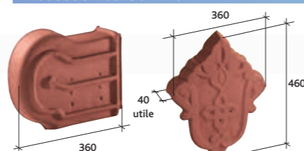
About de rive universelle droit à emboîtement Réf. 1073 (3) Fronton de rive universelle Réf. 1083 (3)
