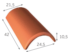
Faitière/arêtier de 42 à recouvrement 2,8 au m 3,5 kg/pièce
