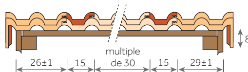
Montage avec tuiles de rives à rabat et demi-tuiles
