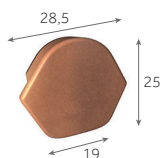
Fronton pour Faitière/arêtier de 42 à recouvrement 2,6 kg/pièce
