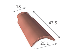
Demi-tuile (utilisation en tuile de couvert pour la finition à l'égout) 2,7 au m 2,6 kg/pièce
