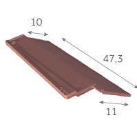
Rive bardelis droite 2,7 au m 2,1 kg/pièce
