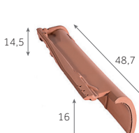
Rive ronde droite 2,5 au m 3,5 kg/pièce
