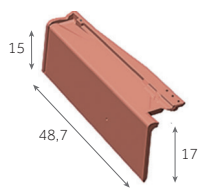
Rive à rabat gauche 2,5 au m 3,3 kg/pièce
