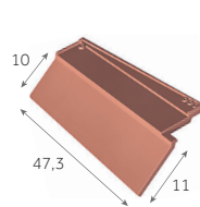
Rive bardelis gauche 2,7 au m 2,1 kg/pièce
