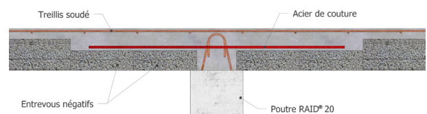
Dispositif C: avec table (3 rangs d'entrevous)
