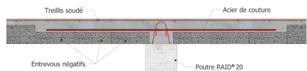
Dispositif C: avec table (3 rangs d'entrevous)
