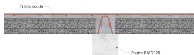
Dispositif A: sans table
