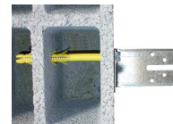
Cheville CQLT-R - vue en coupe dans le parpaing
