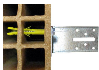
Cheville CQLT-R - vue en coupe dans la brique
