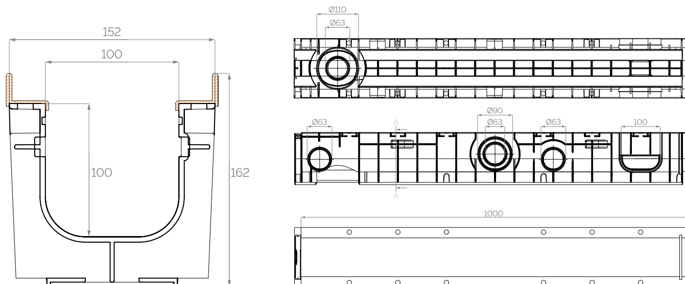
SCHÉMA : CANIVEAU EN PP BORDURE EN ACIER
