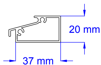
Seuil alu
