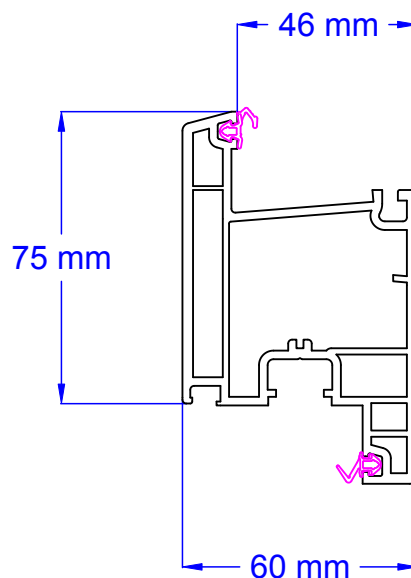
Ouvrant Z 75
