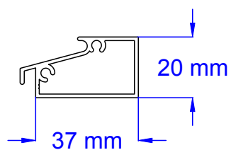
Seuil alu
