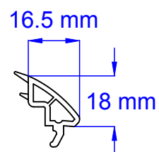
Pareclose 16.5 galbée
