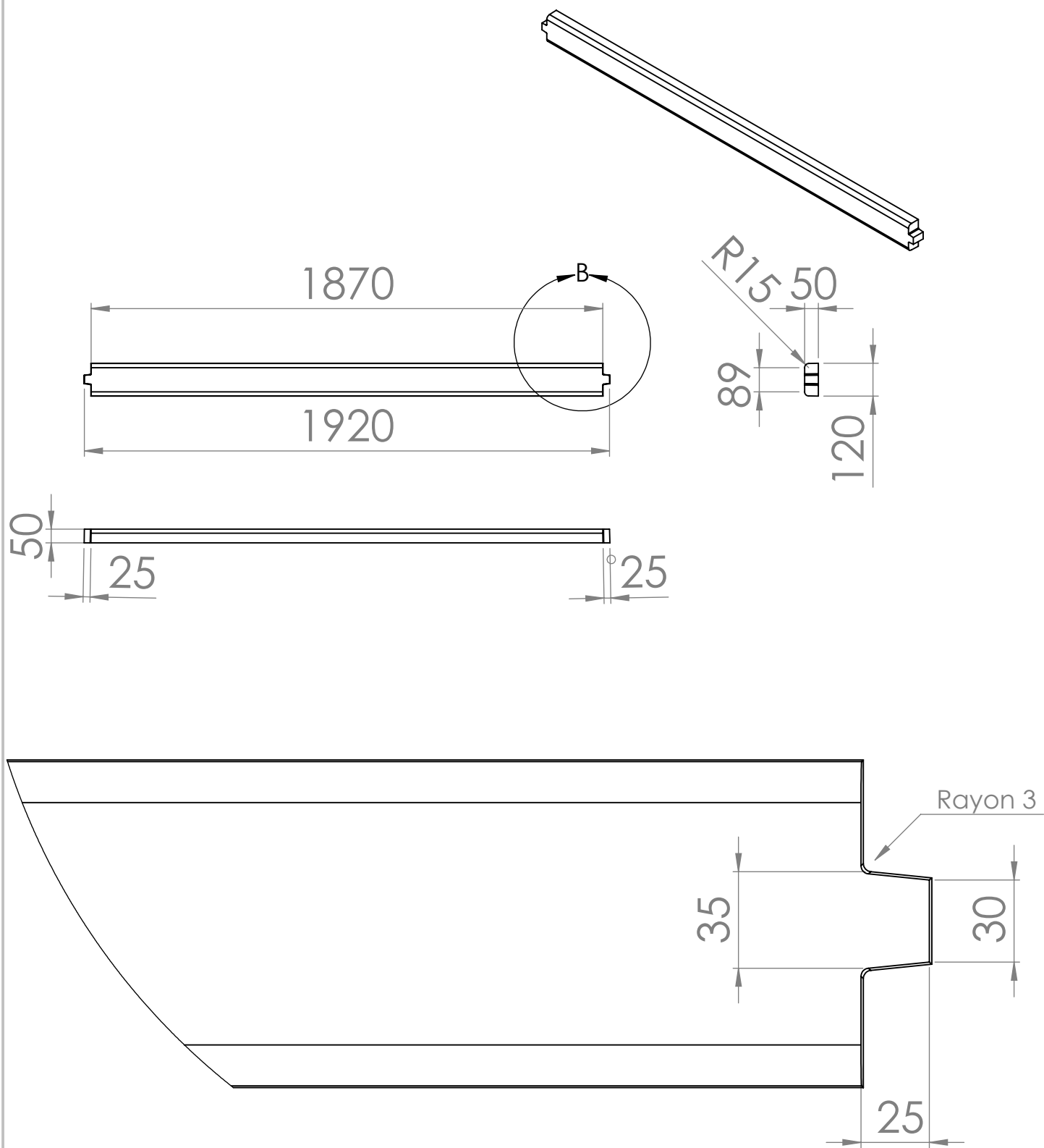
DÉTAIL B ECHELLE 1 : 2
