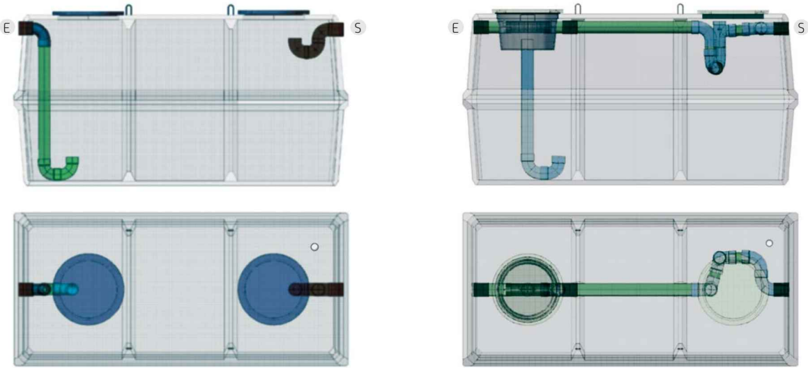
CUVE EN BÉTON ENTERRÉE CUVE EN BÉTON ENTERRÉE AVEC FILTRATION
