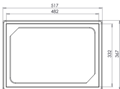
Cadre vue de dessus
