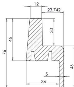
Vue en coupe du cadre
