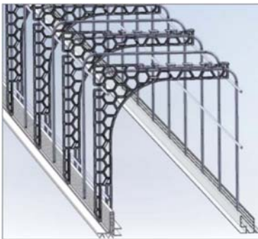
TREILLI RENFORCE
