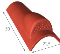
Tuile chatière grillagée (ouverture de 16 cm 2 ) 3,1 kg/pièce
