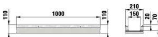
Type 110** fond carré
