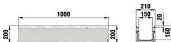
Type 200** fond carré
