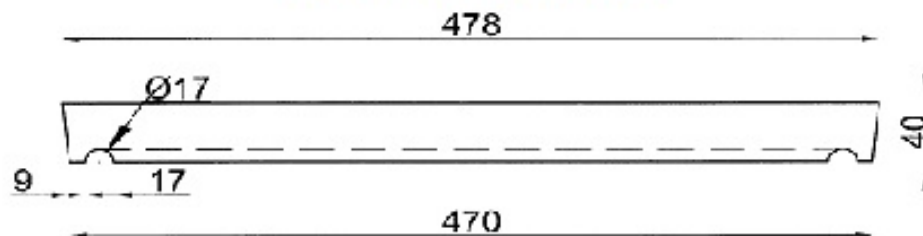
COUVERCLE REGARD 400X400
