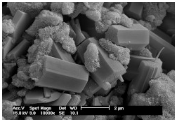
Hydratation d'Ultracolor Plus liant spécial à base de ciment. Noter l'absence de cristaux lamellaires de ciment Portland (hydroxyde de calcium), qui est la cause de l'efflorescence blanchâtre
