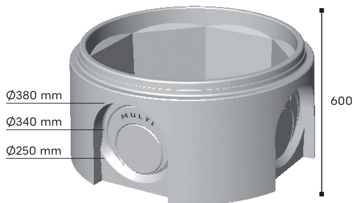
Fonds UNIVERSEL MULTI Ø1000 Réf. CUNVOILE70
