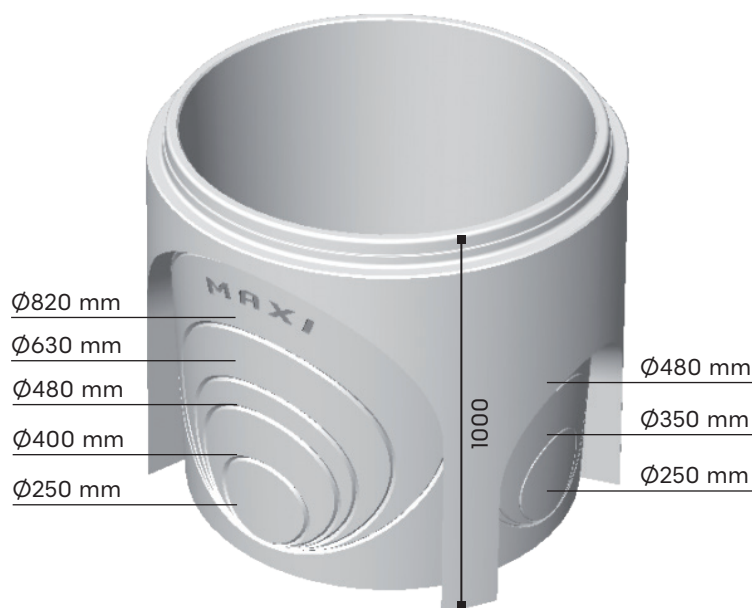
Fonds UNIVERSEL MAXI Ø1000 Réf. CUNVOILE
