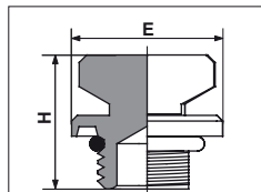
9/S - Bouchon purgeur à joint torique
