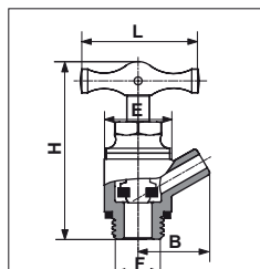
9/D - Robinet purgeur à bec avec vis porte clapet imperdable
