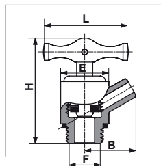
9/E - Robinet purgeur à orifice avec vis porte clapet imperdable
