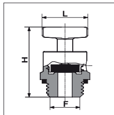
9/G - Purgeur avec écrou porte clapet imperdable
