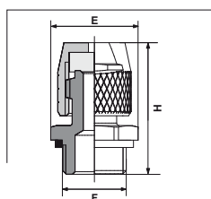
9/S - Bouchon purgeur à joint torique
