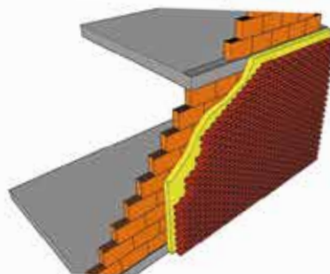
PRINCIPE DE POSE - BGV 15
