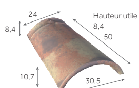
Faîtière/arêtier conique de 50 2,4 au m 4,3 kg/pièce
