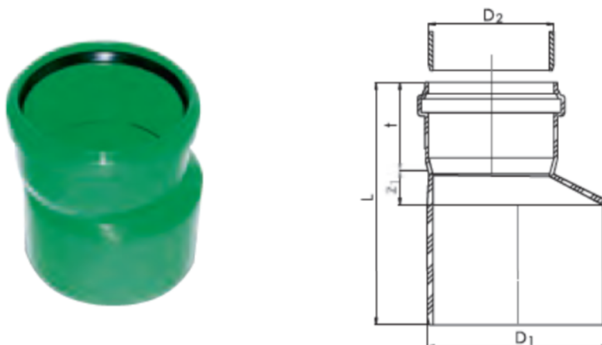
Figure 3.3 : Augmentations excentrées
