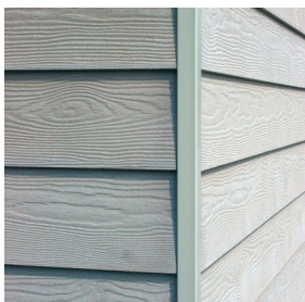
⑥ Travail terminé avec profil d'angle sortant
